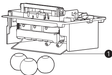
1 Измервателно рамо
